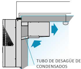
Montaje acaballado (excepto serie 0)
