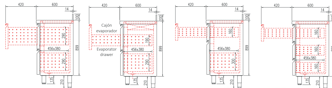
FMR-250 con cajones auto-cierre y motor lado izquierdo opcionales with optionals soft-closing drawers and left side engine
