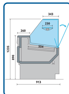
ESQUEMA CRISTAL VERTICAL
