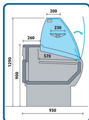
ESQUEMA CRISTAL CURVO
