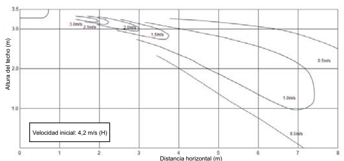
MMC-UP0561HP-E Refrigeración
